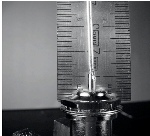
Figure 4.40: La longueur du fil est cruciale.
