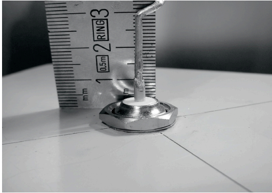
Figure 4.27: La première boucle devrait commencer à 3,0 centimètres de la surface de la plaque.
