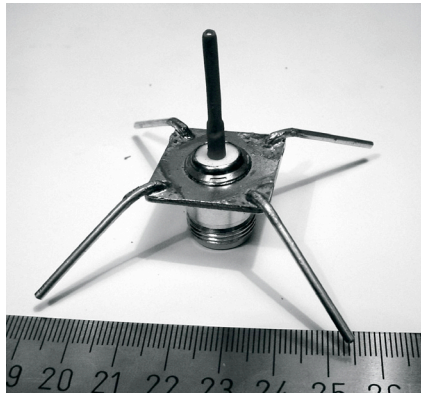
Figure 4.8: Antenne ground-plane d'un quart de longueur d'onde.
