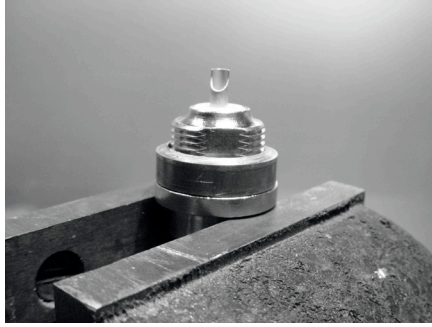
Figure 4.24: Ajouter un tuyau de cuivre comme entretoise aide à obtenir une impédance d'antenne de 50 Ohms.
