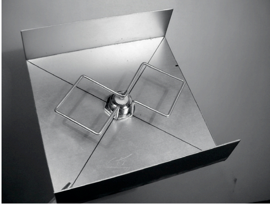
Figure 4.12: Une BiQuad.
