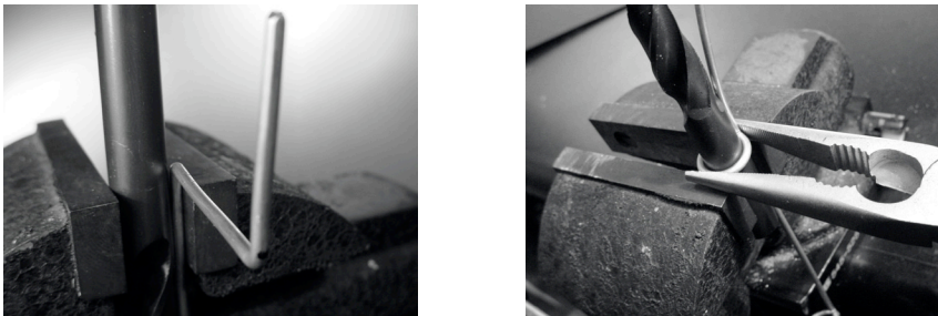
Figure 4.18: Courber le fil autour de la perceuse pour faire une boucle.
