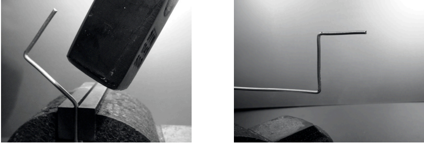
Figure 4.17: Plier le fil en forme de « Z ».
