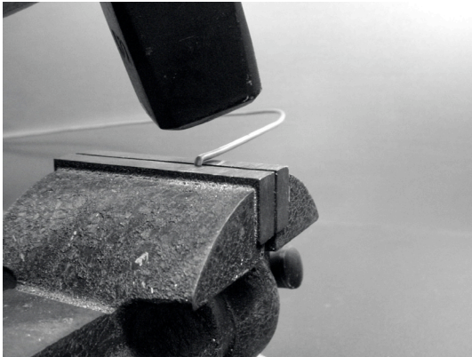
Figure 4.16: Frapper doucement sur le fil pour faire une courbe fermée.
